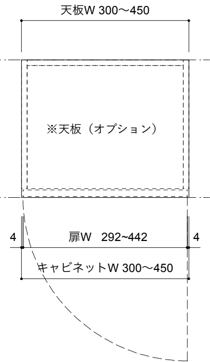
平面図
