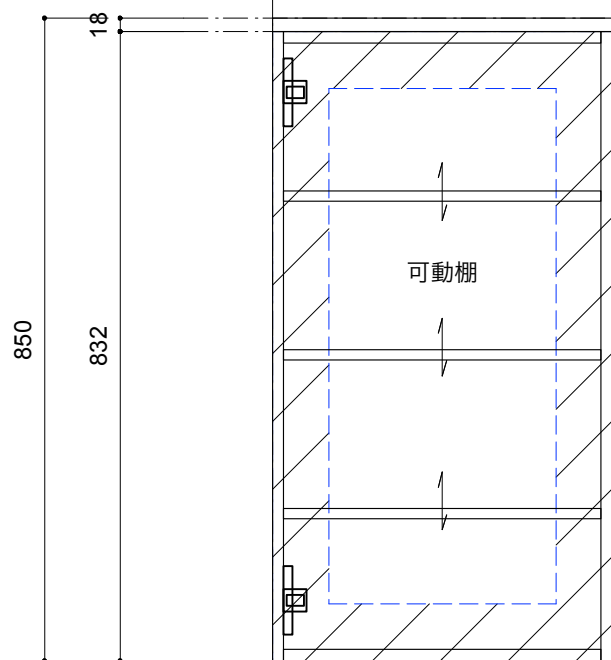
左吊り元仕様
