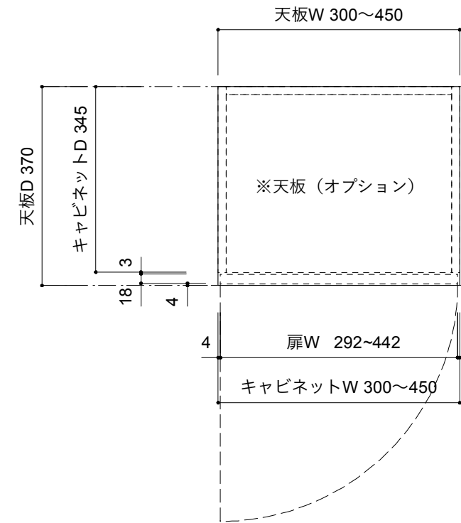
平面図
