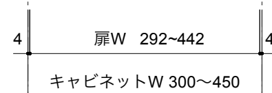
左吊り元仕様
