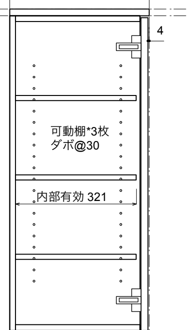
断面図
