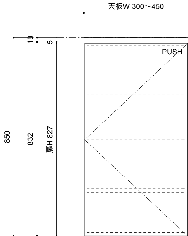
正面図
