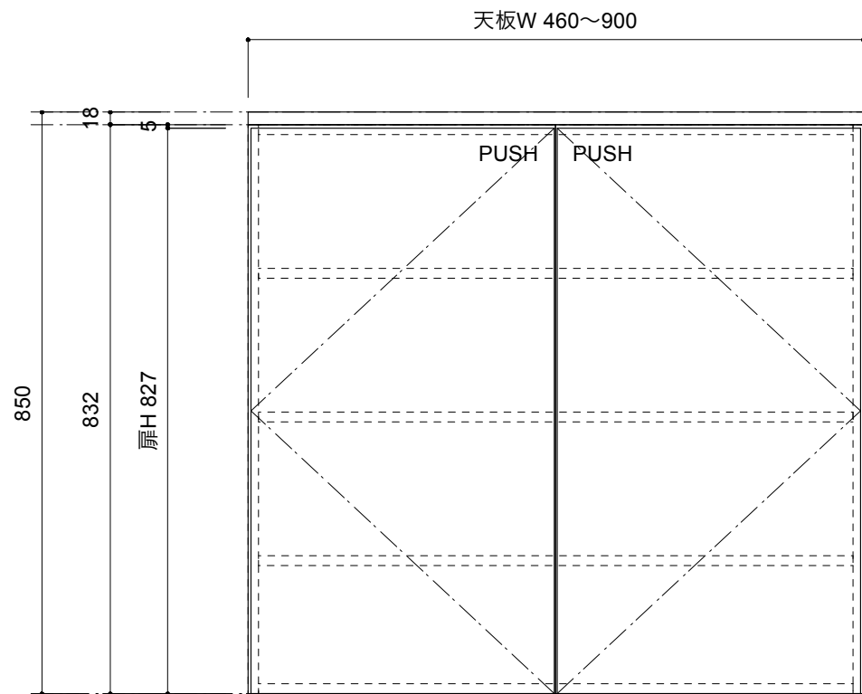
正面図
