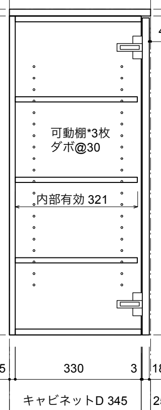
断面図
