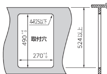
取付開口寸法
