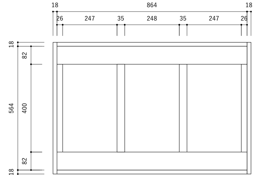
背面図
