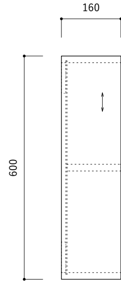
側面図-2段
