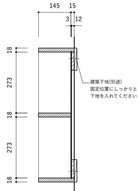
断面図-2段
