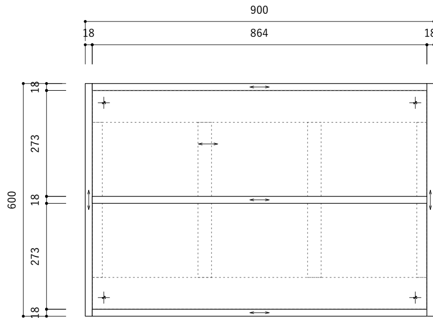
正面図-2段
