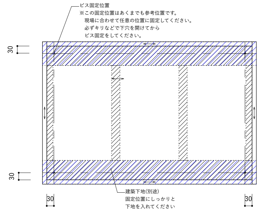
固定用ビス位置(参考)
