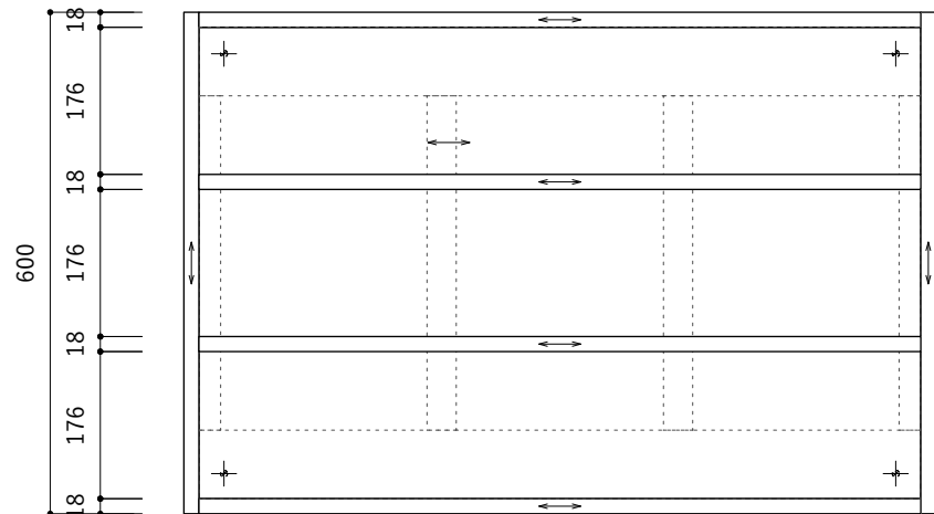
正面図-3段
