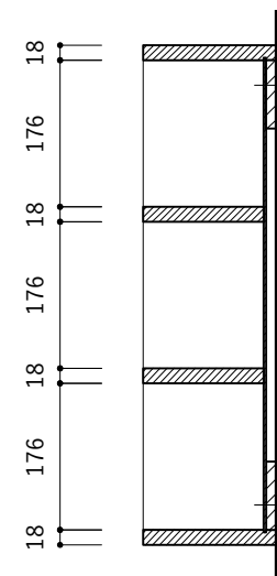
断面図-3段
